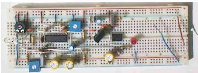
Prototipo realizzato su bread board
