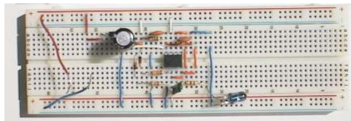
Prototipo realizzato su bread board
